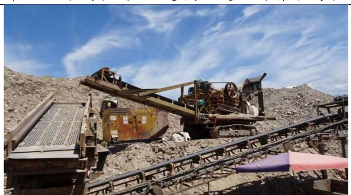
114年4月17日先經震動篩，再使用破碎機(違反作業程序)
