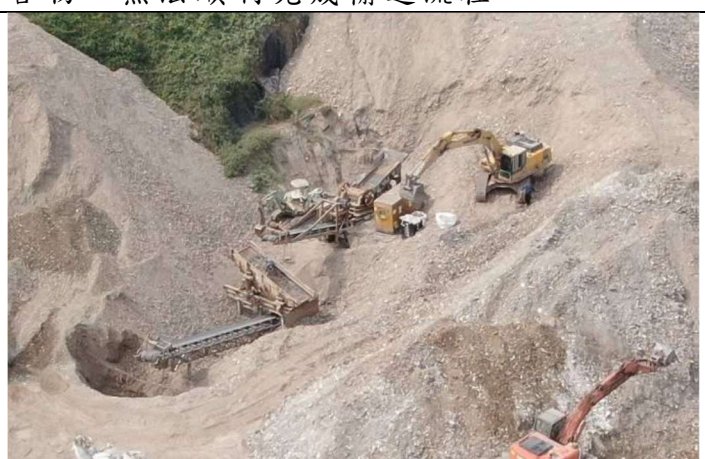
114年2月19日由左而右為輸送帶、震動篩、破碎機(缺少磁選機，違反作業程序)
