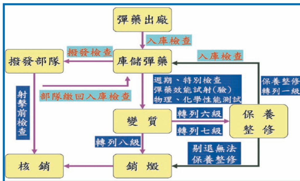
圖1 彈藥壽期管理技術檢查
