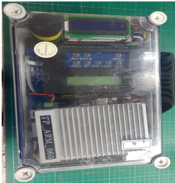
圖5 輻射監測器(加馬偵檢器)
