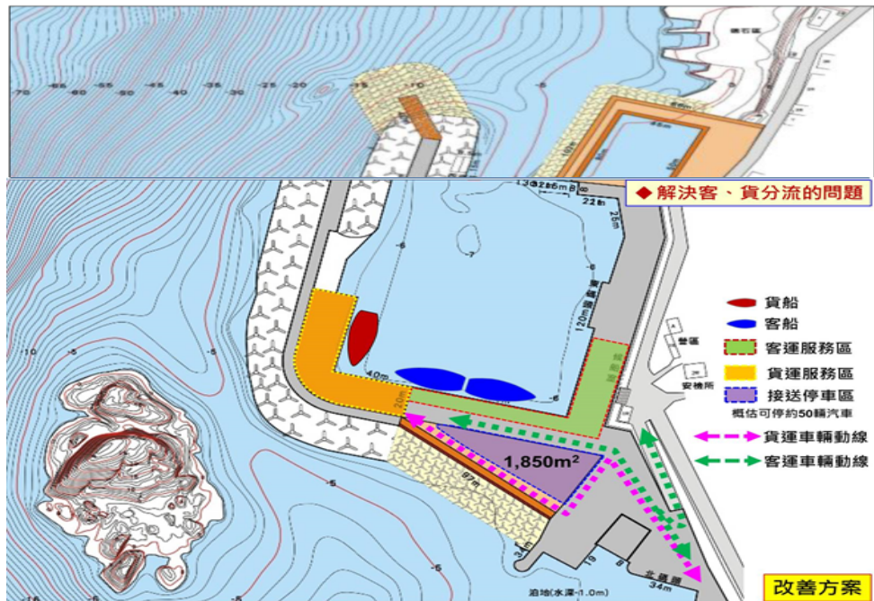
圖3 蘭嶼開元港現況及改善方案配置圖
