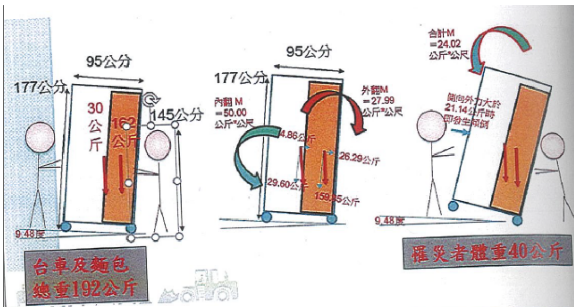
圖2 模擬計算高度177公分麵包台車僅需21.4公斤推力即會傾倒。
