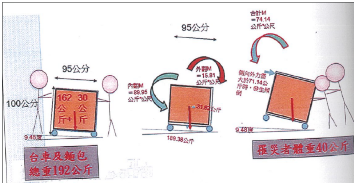
圖3 模擬計算高度100公分麵包台車則僅需71.4公斤推力方能傾倒。 資料來源：新北勞檢處重大職災報告書。
