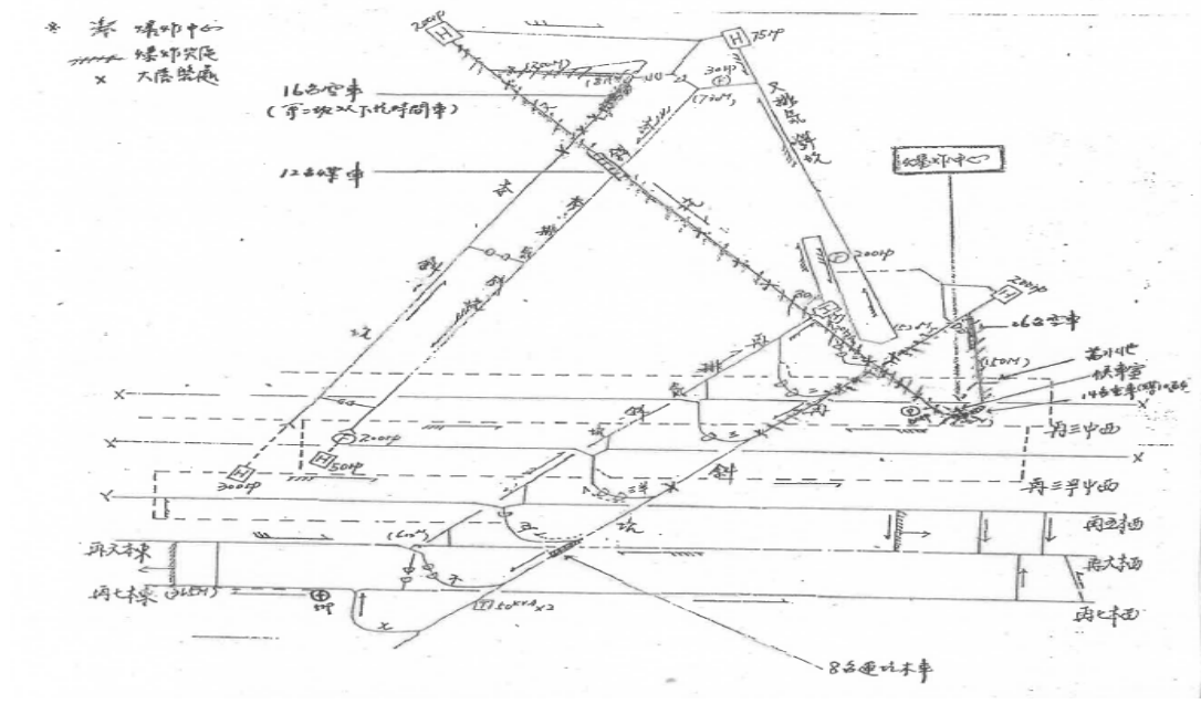
圖6 海一煤礦災變地點略圖
