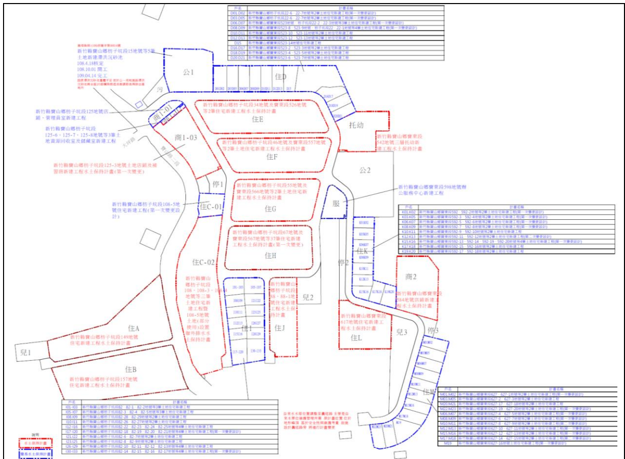
圖3、本案水土保持概況圖
