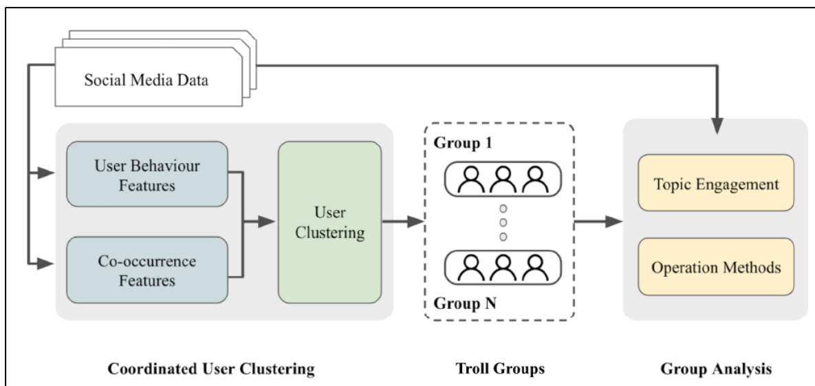
圖2. 社群網路協同行為分析流程概要(資料來源：Taiwan AI Labs)
