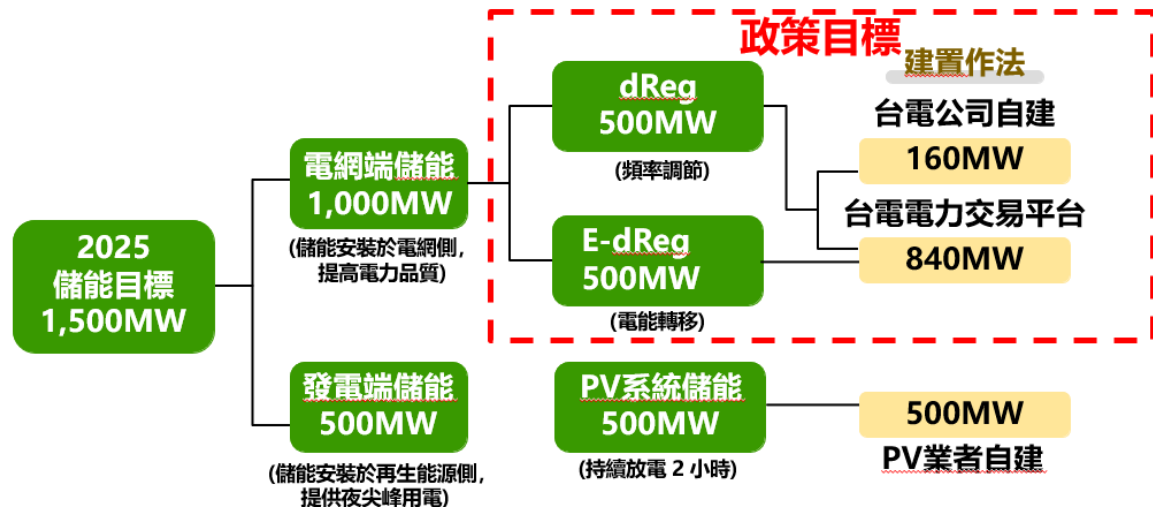
圖10 台電公司儲能目標1,500MW(2025年)
