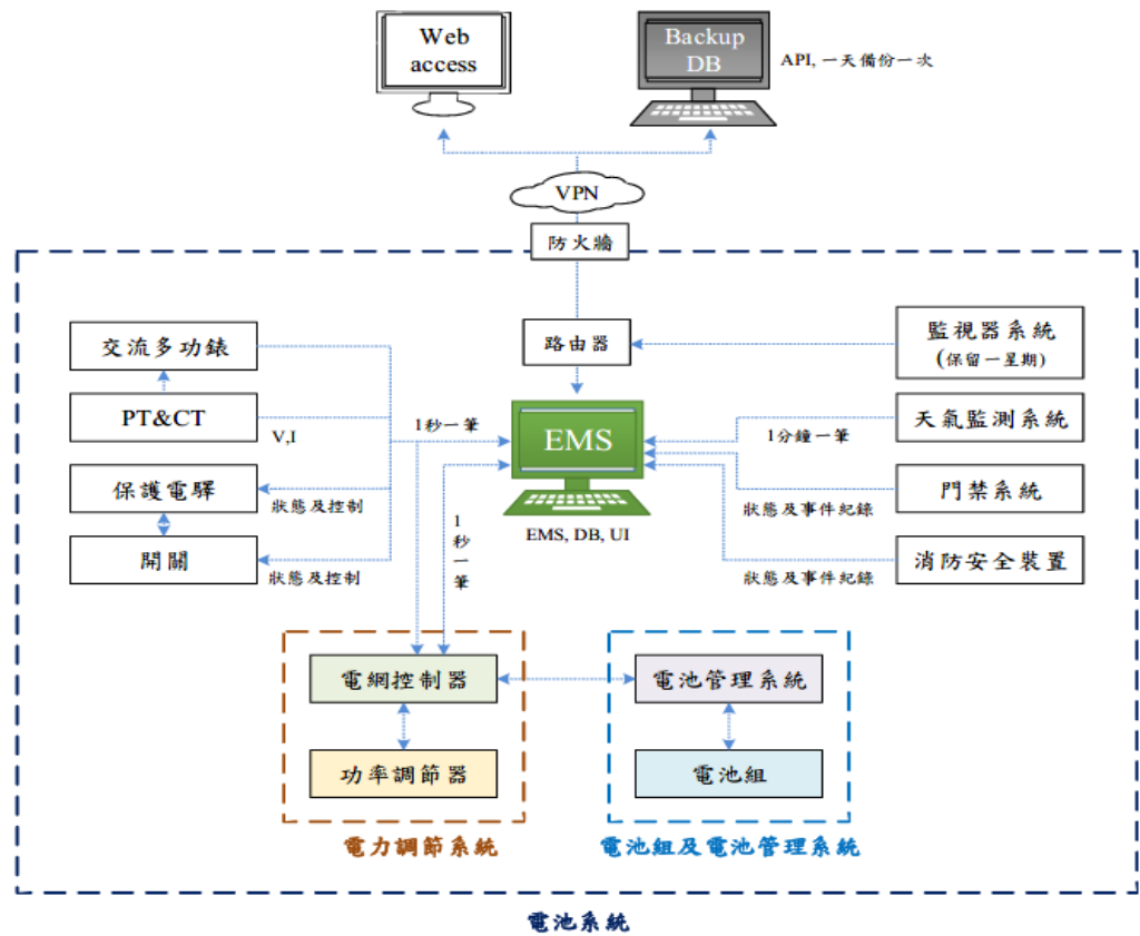
圖8 併網功能驗證系統資通訊流示意圖
