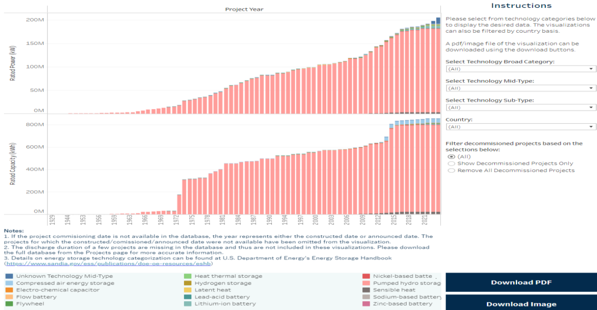
圖1 全球儲能累計額定功率、額定容量統計(~2023)
