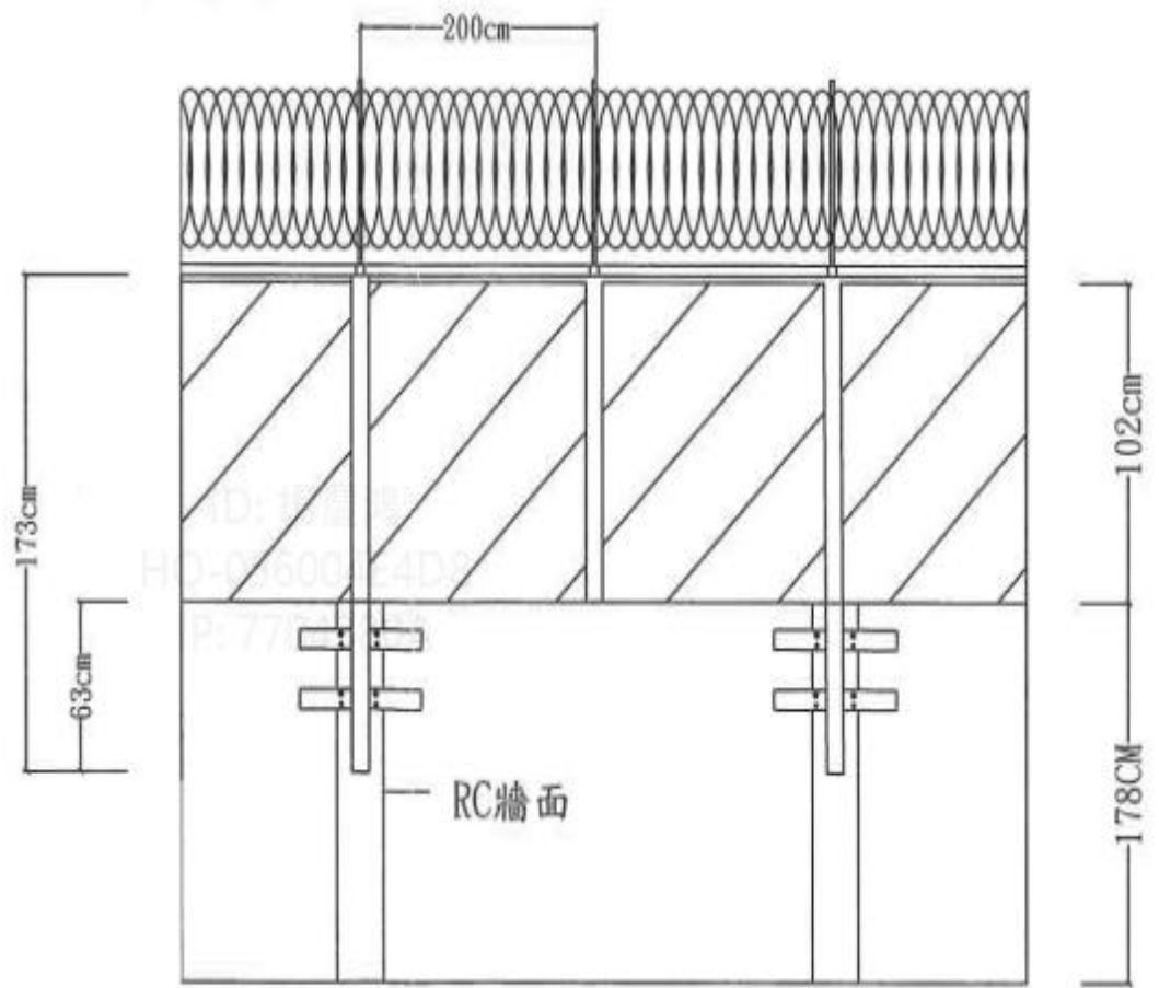
圖1 隔音牆建置評估圖(資料來源：空軍第○聯隊113年11月29日履勘簡報資料：考量新購戰機預計○○年底進駐志航機場，後續噪音範圍影響更甚，為達有效之防制，擬評估隔音牆建置之可行性)
