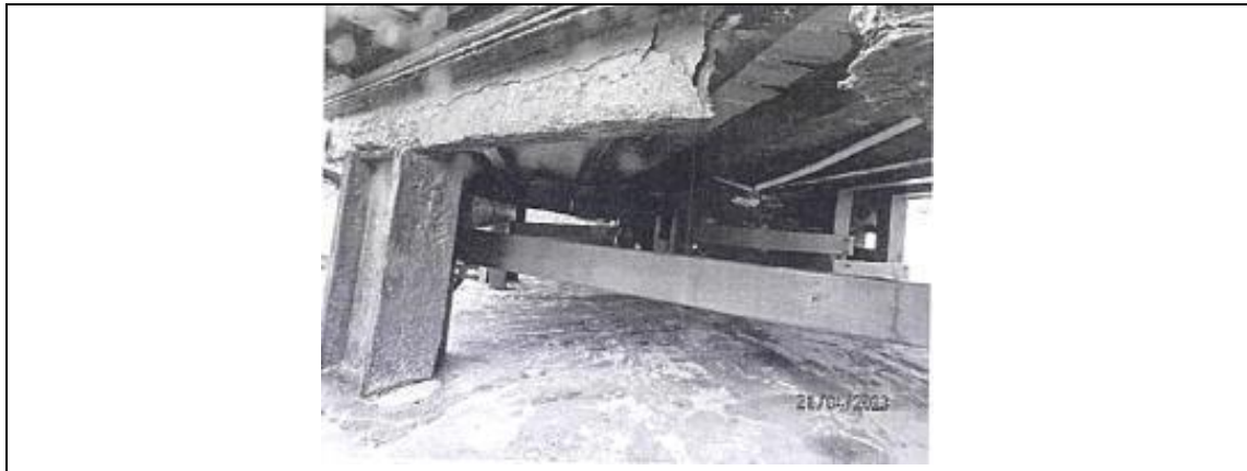
圖2 野柳地質公園景觀橋及木棧道（R木棧道）橋梁下部現況照片 資料來源：111-112年北觀管理處轄管橋梁及構造物巡檢工作委託技術服務案，第4次定期檢測成果報告書。
