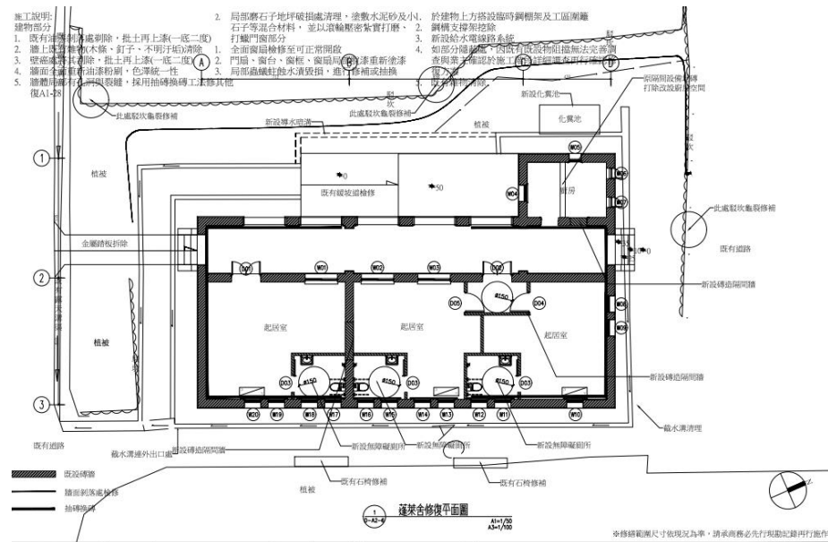
圖 蓬萊舍修復平面圖
