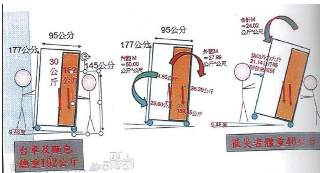
圖2 模擬計算高度177公分麵包台車僅需21.4公斤推力即會傾倒。
