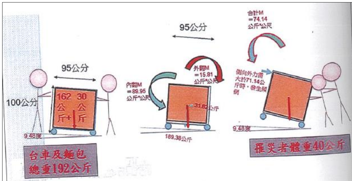
圖3 模擬計算高度100公分麵包台車則僅需71.4公斤推力方能傾倒。
