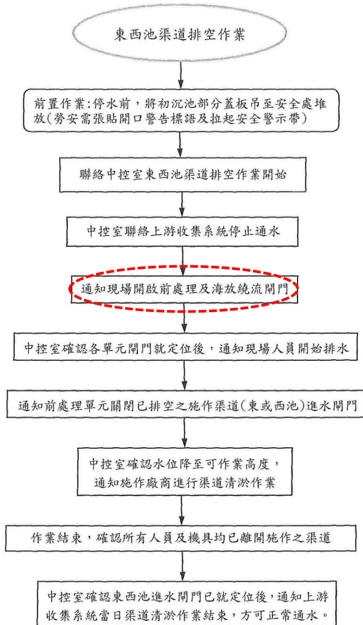
排水作業流程圖
